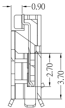
剖面 A-A
